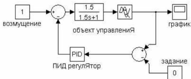
Рисунок 1 – Модель одноконтурной системы автоматического регулирования
