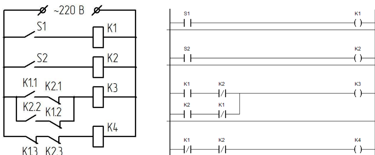
Рисунок 2 – Релейно-контактная схема и ее аналог на языке LD
