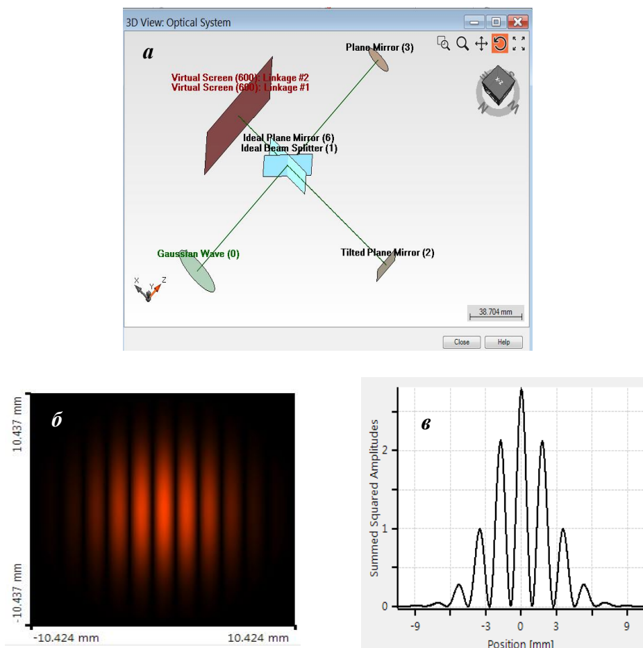
Рисунок 1 – а – 3D схема интерферометра Майкельсона; б – интерференционная картина на виртуальном экране (длина волны лазерного излучения \lambda=632\text{nm} ); в - распределение интенсивности света в интерференционной картине
