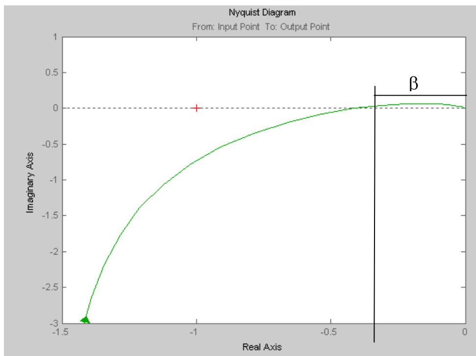
Рисунок 2 – График АФЧХ для системы с ПИ-регулятором
