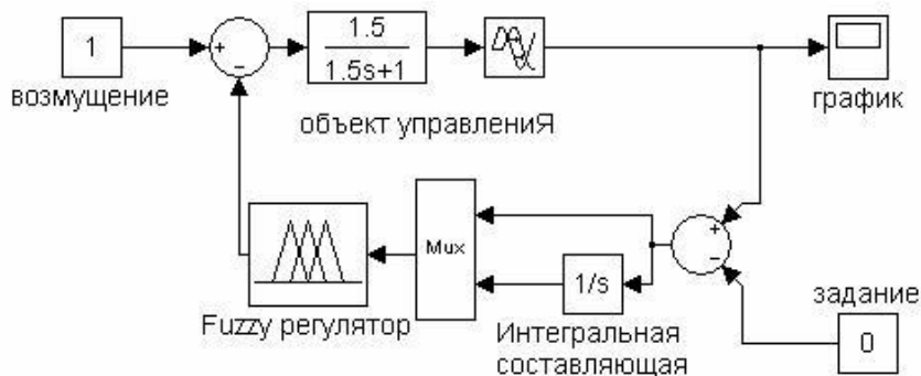
Рисунок 2 – Модель одноконтурной системы автоматического регулирования с ПИ-подобным fuzzy-регулятором
