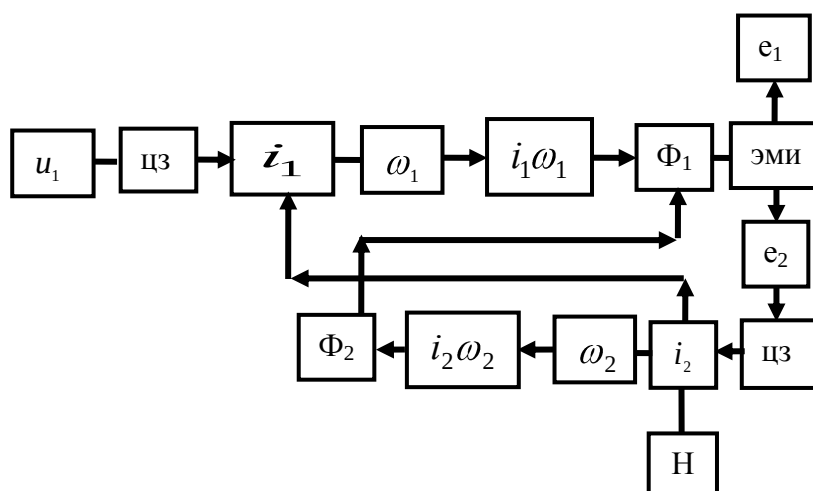
Рисунок 1 – Условно - логическая схема работы трансформатора под нагрузкой
