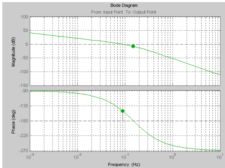
Рисунок 1 – Графики ЛАФЧХ системы с ПИ-регулятором
