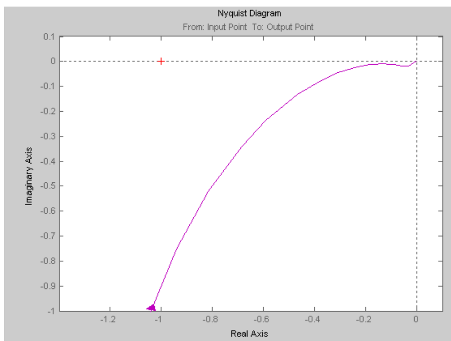
Рисунок 4 – График АФЧХ для системы с ПИД-регулятором
