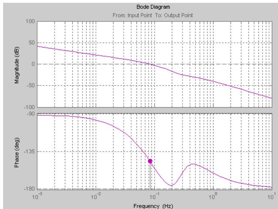
Рисунок 3 – Графики ЛАФЧХ системы с ПИД-регулятором
