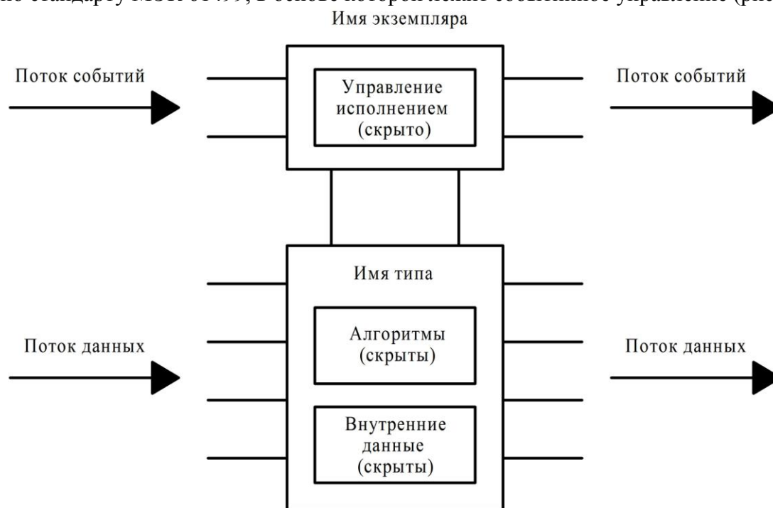
Рисунок 1 – Функциональный блок стандарта МЭК 61499
