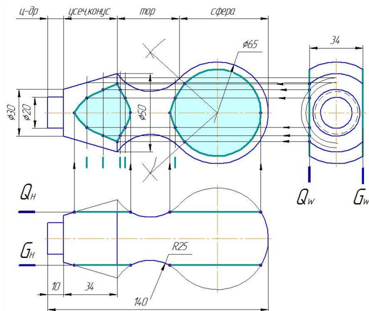
Рисунок 2 – Выполнение графической работы по построению линий среза на детали
