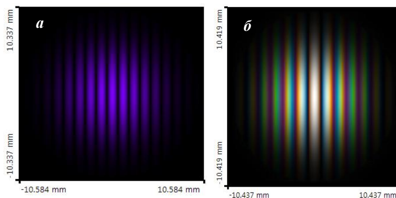
Рисунок 2 – а – изменение ширины интерференционной картины (длина волны светового излучения \lambda=435 нм); б – реализация триплета длин волн (473 нм, 532 нм, 635 нм)
