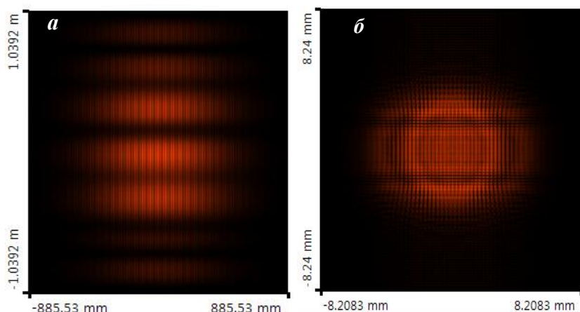
Рисунок 3 – Дифракция световой волны на синусоидальной дифракционной решетке: а – дифракция плоской волны; б дифракция сферической волны
