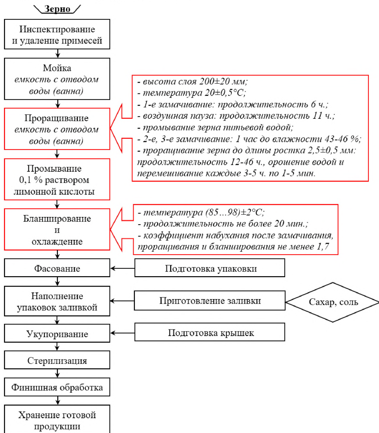
Рисунок 9 – Технологический процесс производства консервов «Зерна пророщенные (пшеница)»
