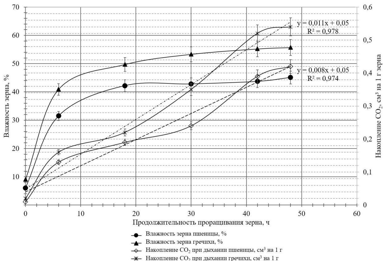
Рисунок 4 – Влияние проращивания на изменение влажности и накопление \text{CO}_2 при дыхании зерна пшеницы и гречихи
