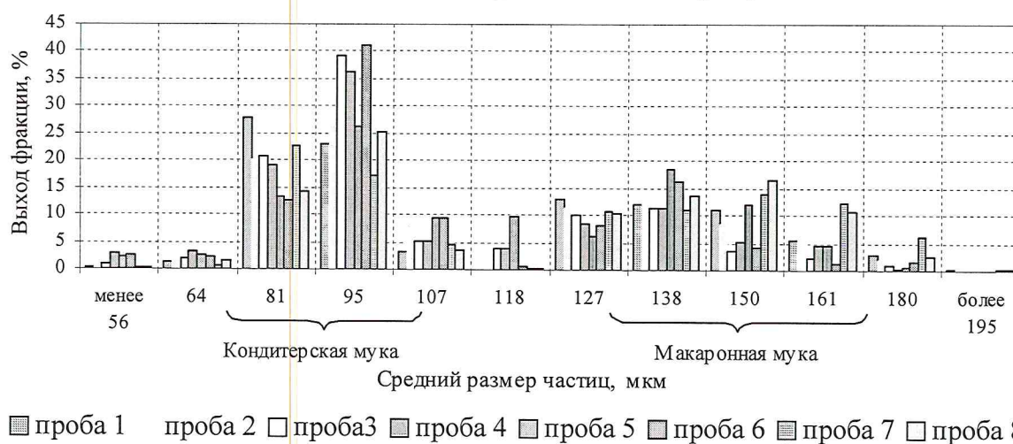
Рисунок 1 – Гранулометрический состав тритикалевой муки
